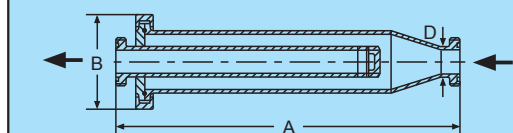
螺式直通过滤器 型号type: IG06-R
