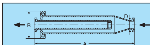
卡式直通过滤器 型号type: IG06-K
