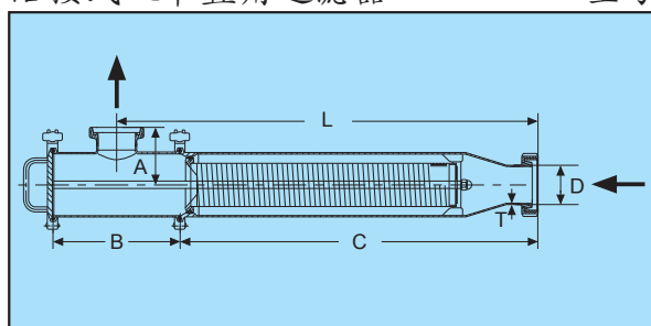
磁性过滤器
