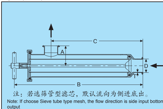
直角过滤器
