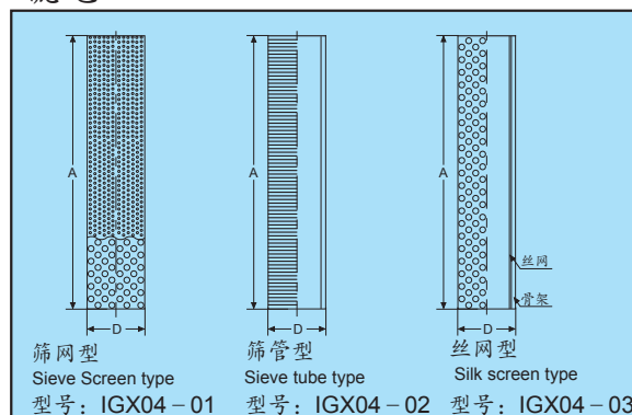
滤芯
