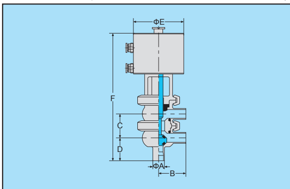
TT型气动截止阀
