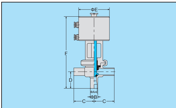
LL型气动截止阀
