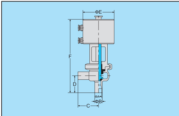
T型气动截止阀
