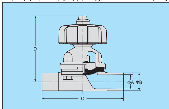
卡式手动隔膜阀(锻造)
