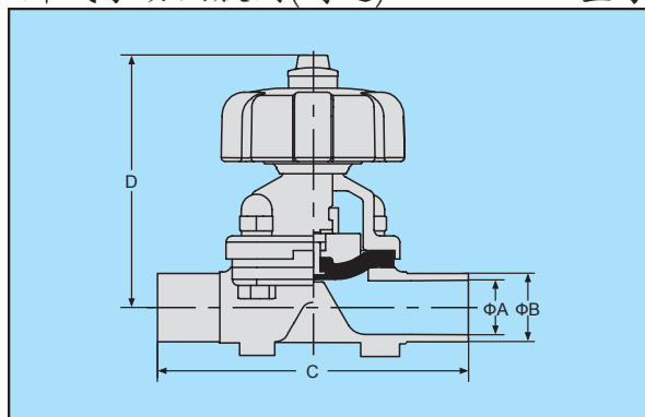
卡式手动隔膜阀(铸造)
