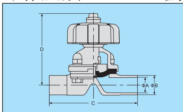
卡式手动隔膜阀
