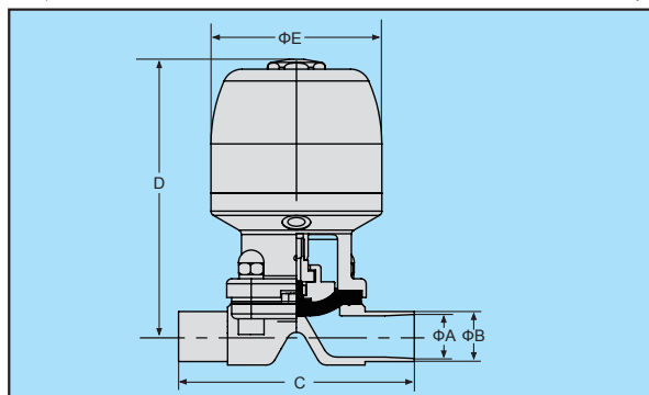
卡式气动隔膜阀
