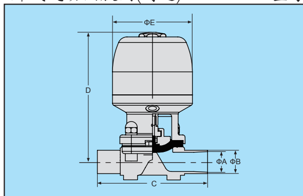
卡式气动隔膜阀(铸造)
