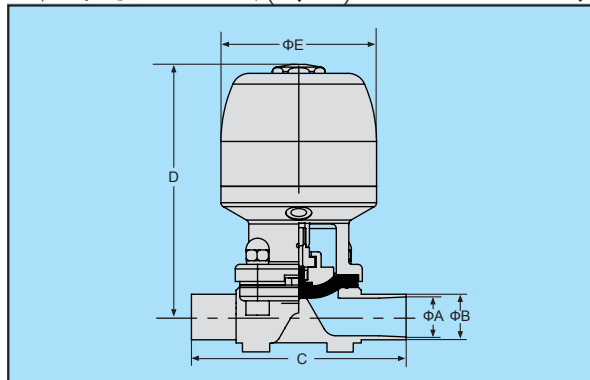
焊式气动隔膜阀(铸造)
