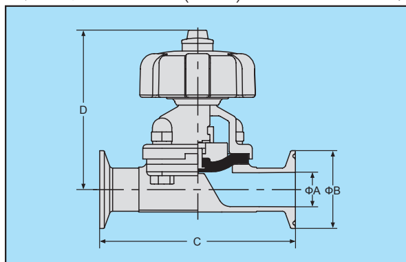
焊式手动隔膜阀(锻造)
