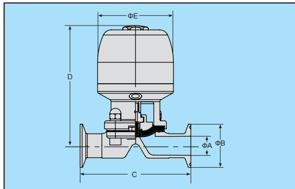
焊式气动隔膜阀
