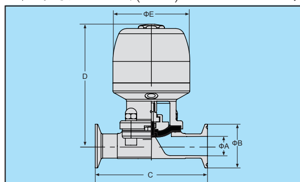
卡式气动隔膜阀(锻造)
