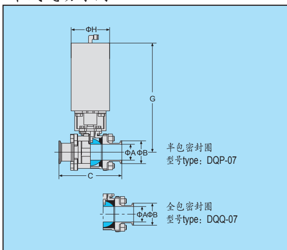
卡式气动球阀
