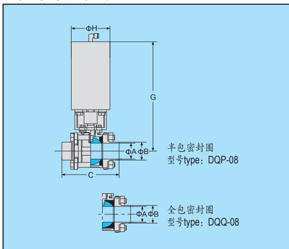
焊式气动球阀
