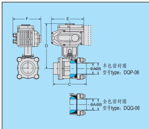
焊式电动球阀
