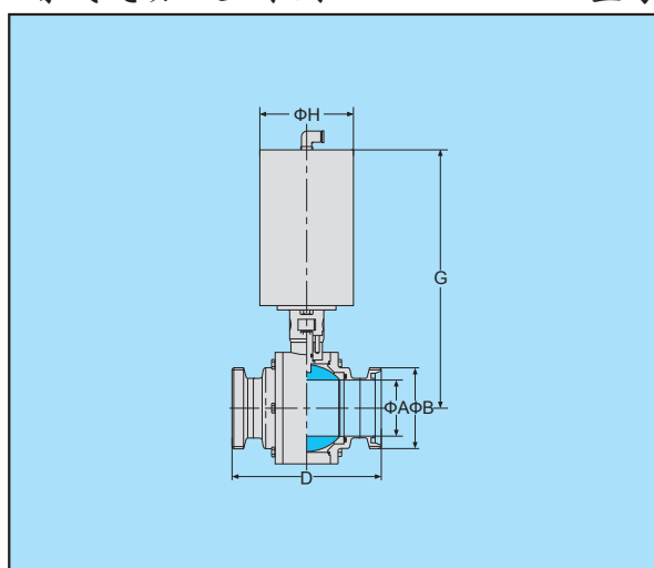
螺式气动卫生球阀
