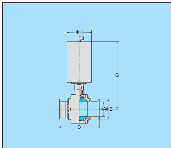
焊式气动卫生球阀
