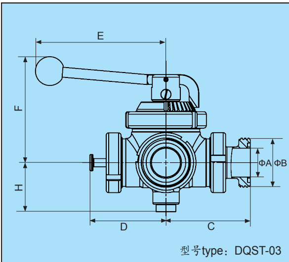
螺式手动三通球阀
