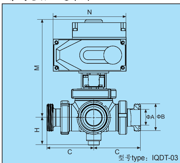
螺式电动三通球阀
