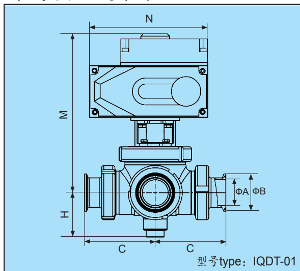
螺式电动三通球阀
