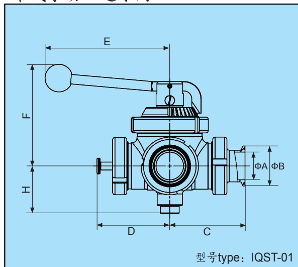
螺式手动三通球阀
