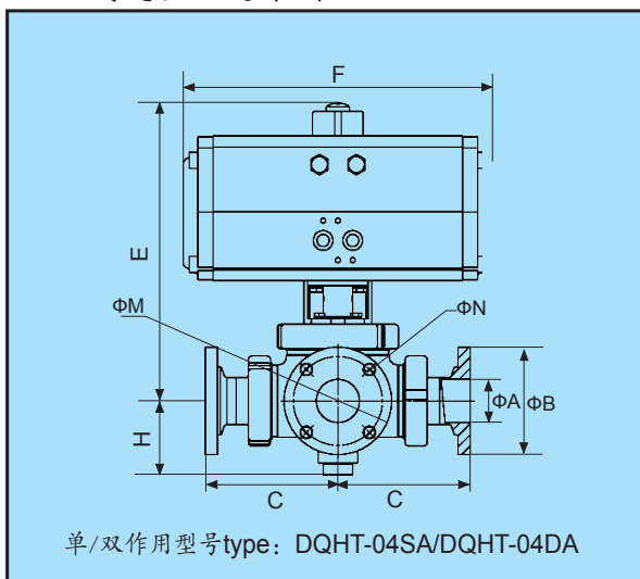
法兰式气动三通球阀
