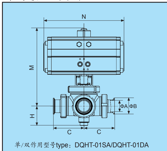
卡式气动三通球阀
