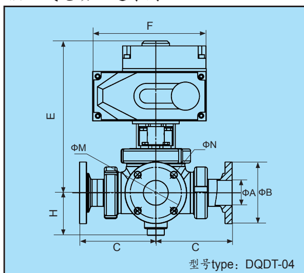
法兰式电动三通球阀
