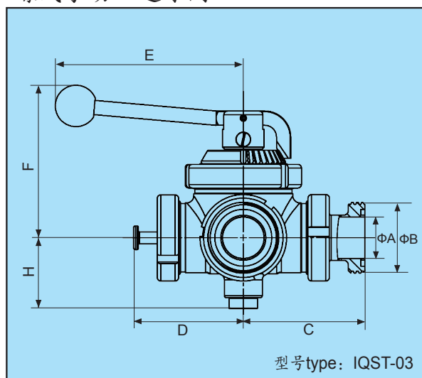
法兰式手动三通球阀
