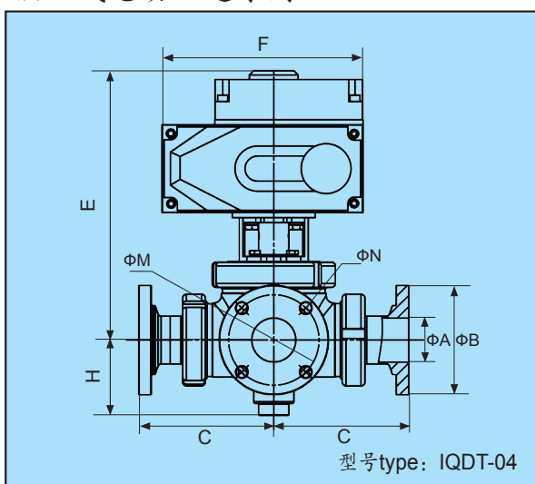
法兰式电动三通球阀
